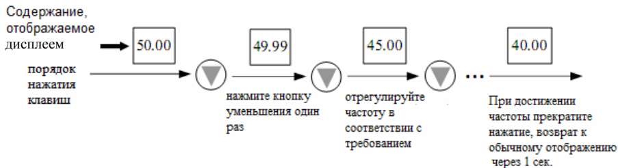
Рис. 4-8 Пример регулировки установленной частоты
