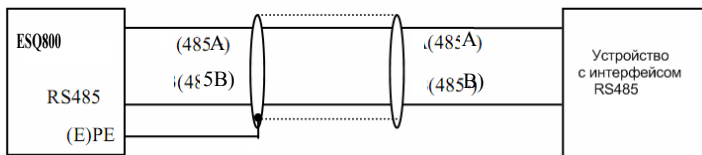
Рис. 3-11 Подключение проводов клеммной коробки связи
