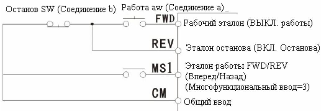
Пример прокладки проводов 3-проводной системы
